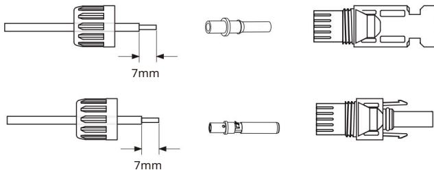
Imaginea 3.3 Dezasamblați piulița cu cap a conectorului
