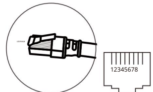
Port Modbus
